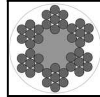
6X7 EN12385-4 JUS C.H1.070 DIN 3055
