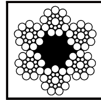
6X19 seale=6X(1+9+9) FC
