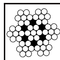
6X7=6X(1+6) IWRC EN12385-4 JUS C.H1.070 DIN 3055
