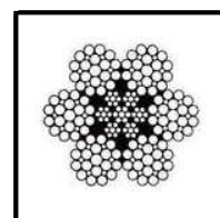
6X19 Filler=6X(1+6+6F+12) IWRC EN12385 JUS C.H1.086 DIN 3057
