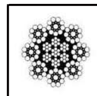
8X19 Seale=8X(1+9+9) IWRC
