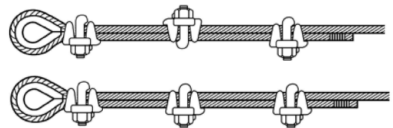
Neppravilno Postavljanje Stega za Čelično Uže
